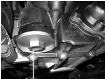
Tappo filtro a cartuccia (7)
