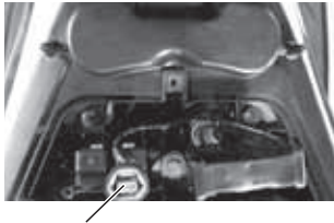
Connettore di diagnosi
