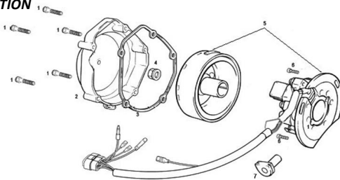
ENCENDIDO IGNITION
