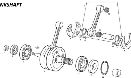
CIGÜEÑAL CRANKSHAFT
