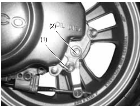
(1) Vite di drenaggio (2) Vite di ispezione
