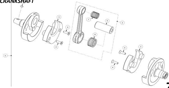
CIGÜEÑAL CRANKSHAFT
