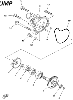
BOMBA AGUA WATER PUMP
