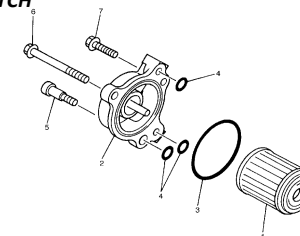
EMBRAGUE CLUTCH
