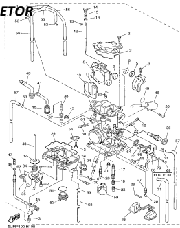
CARBURADOR CARBURETOR
