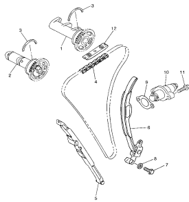
ÁRBOL DE LEVAS CAMSHAFT & CHAIN
