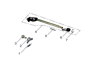
MECANISMO DE CAMBIO GEARSHIFT MECHANISM
