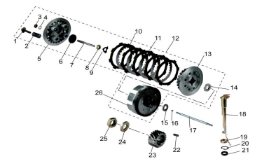
EMBRAGUE CLUTCH
