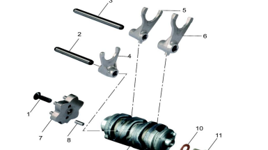
MECANISMO DE CAMBIO GEARSHIFT MECHANISM
