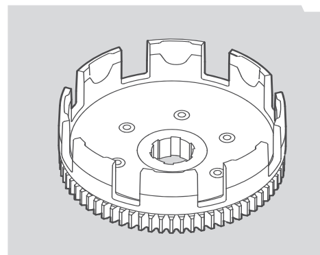
CLOCHE D'EMBRAYAGE CLUTCH BELL
