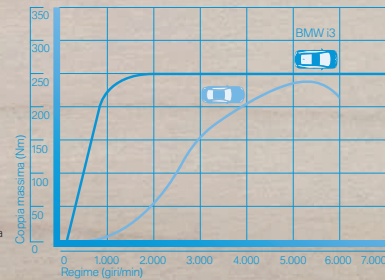
Grafico della curva di coppia.
