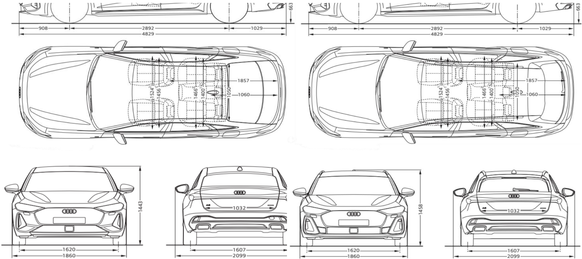
Misure in millimetri (indicazione delle dimensioni con massa a vuoto) 1 Larghezza al livello delle spalle 2 Larghezza al livello dei gomiti 3 Spazio massimo per la testa
