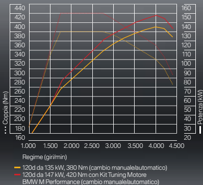
Valori di potenza e coppia della BMW 120d con Kit Tuning Motore BMW M Performance Pieno carico 120d
