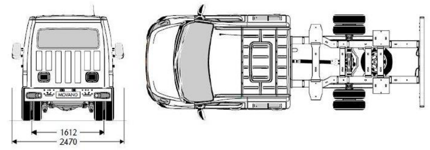
*1575 Esclusa la traversa posteriore
