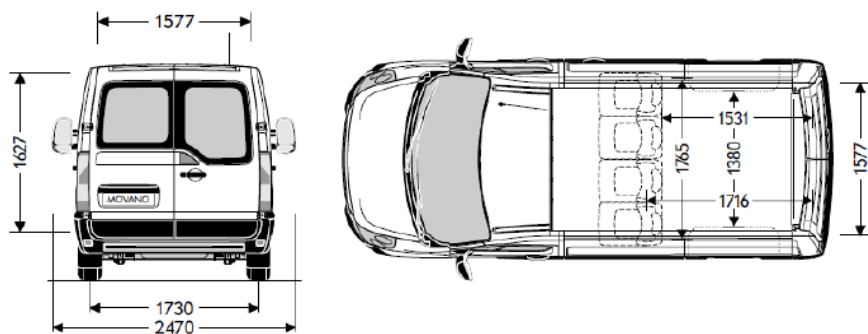
Furgone Doppia Cabina L1H1 – T. Anteriore
