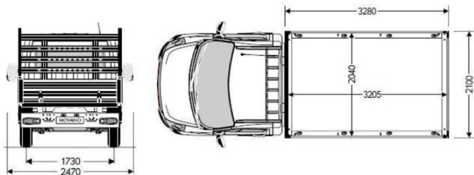
Ribaltabile - L2 – T. Anteriore
