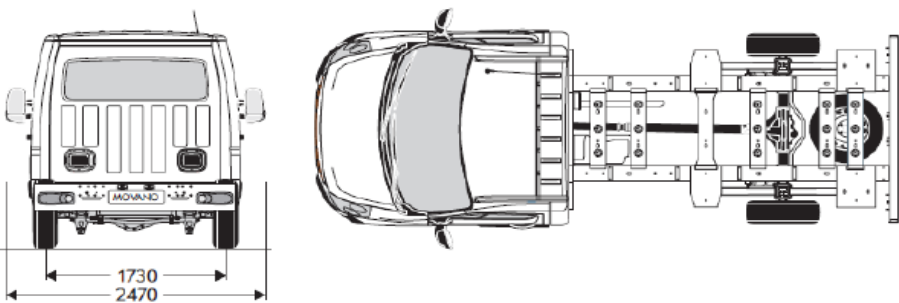
L2 – T. Posteriore
