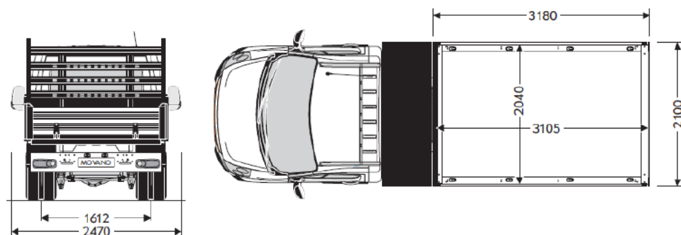
Ribaltabile - L3 – T. Posteriore Gemellato
