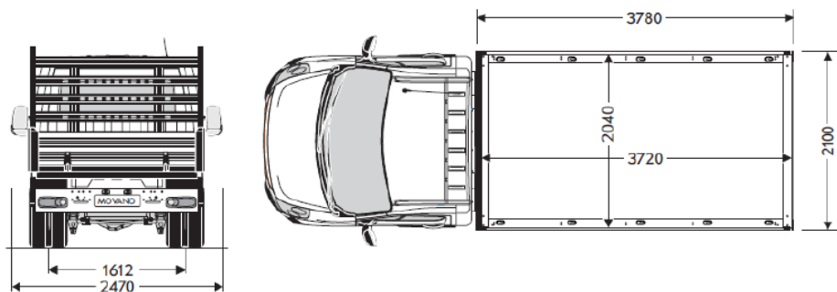
Fisso - L3 – T. Posteriore Gemellato
