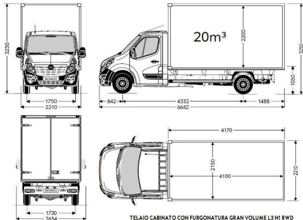
Furgonato - L3 – T. Posteriore
