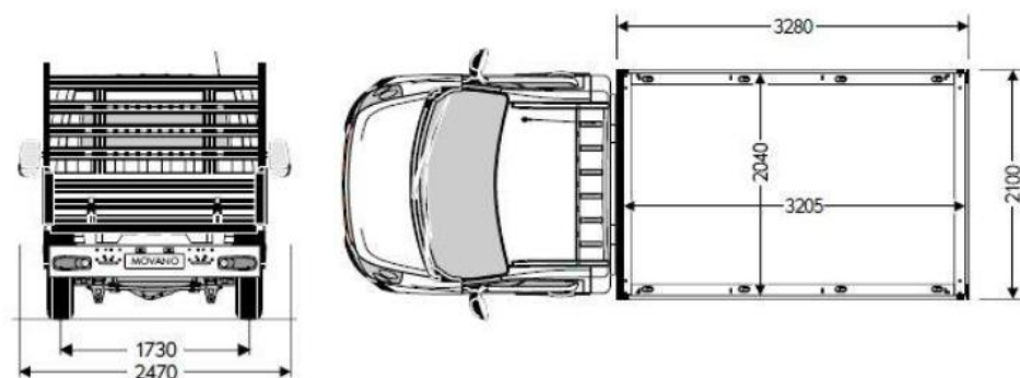
Ribaltabile - L2 – T. Posteriore
