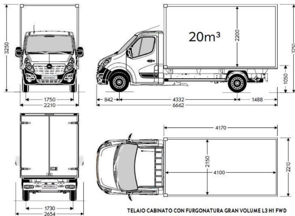
Furgonato - L3 – T. Anteriore
