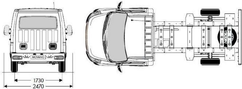
L2 – T. Anteriore
