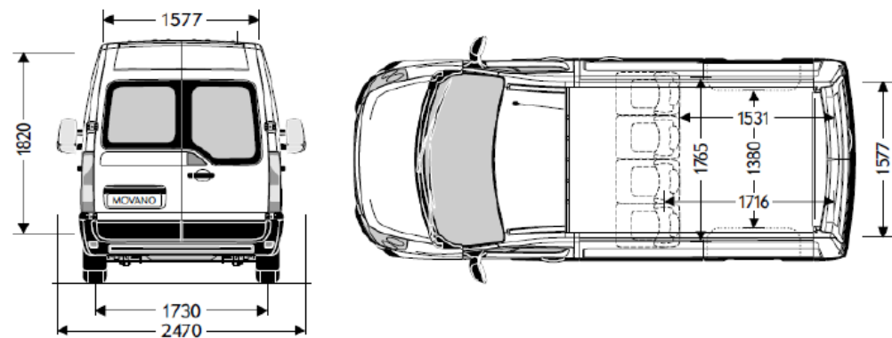
Furgone Doppia Cabina L1H2 – T. Anteriore
