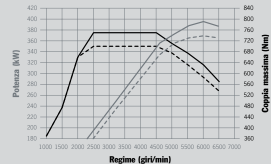
— Cayenne Turbo con kit di potenziamento - - - - - Cayenne Turbo di serie
