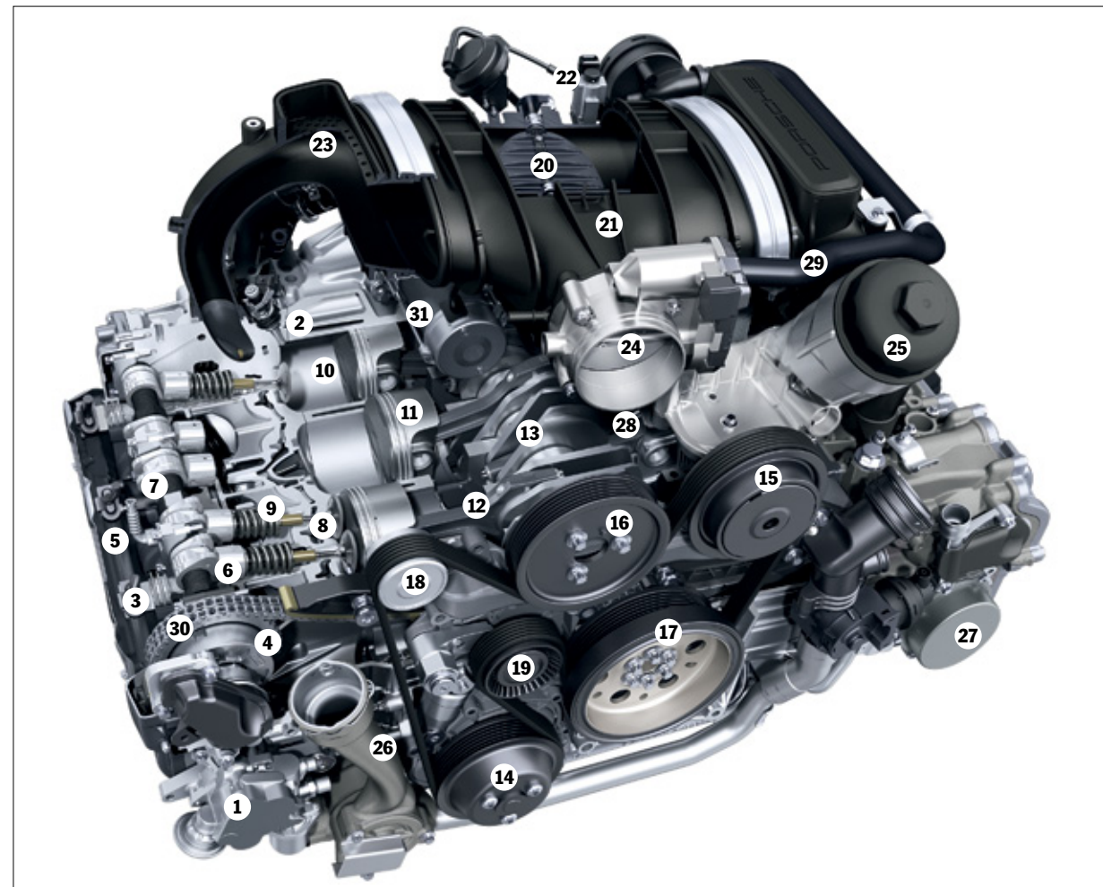
Motore boxer da 3,8 litri
