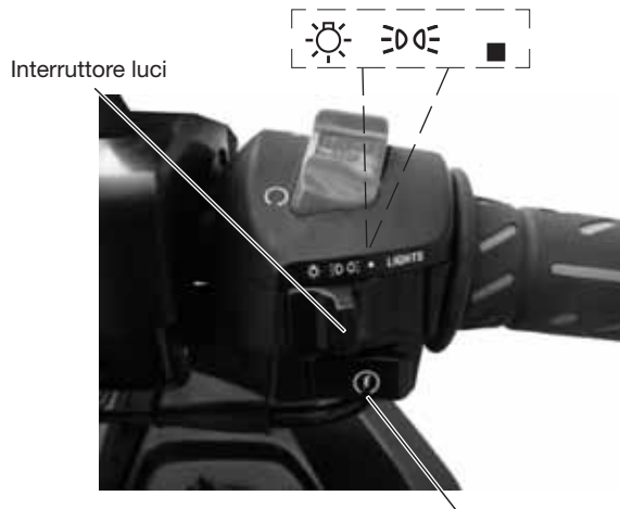
Segnalazione di emergenza (Hazard) Pulsante avviamento
