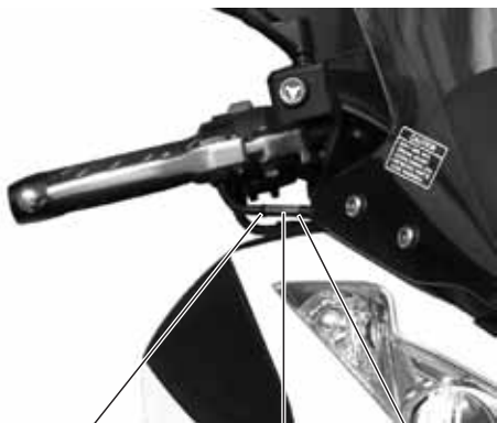
Controdado (3) Vite di regolazione (2) Manicotto in gomma (1)
