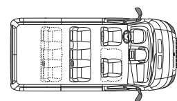
Combi vetrato 5/6 - 8/9 posti
