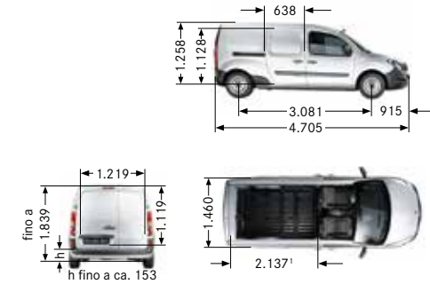
Furgone Extralong con passo 3.081 mm
