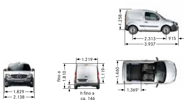
Furgone Compact con passo da 2.313 mm
