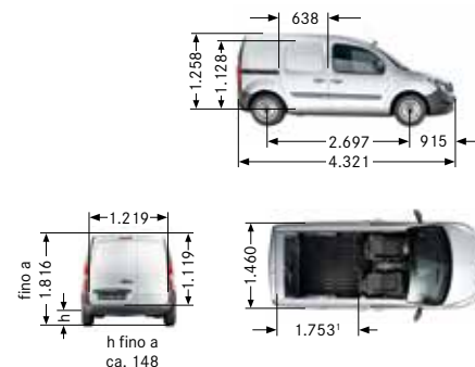
Furgone Long con passo da 2.697 mm
