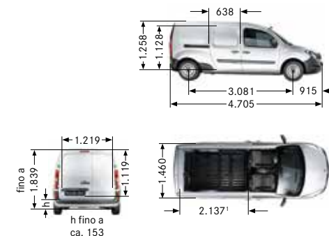
Furgone Extralong con passo da 3.081 mm
